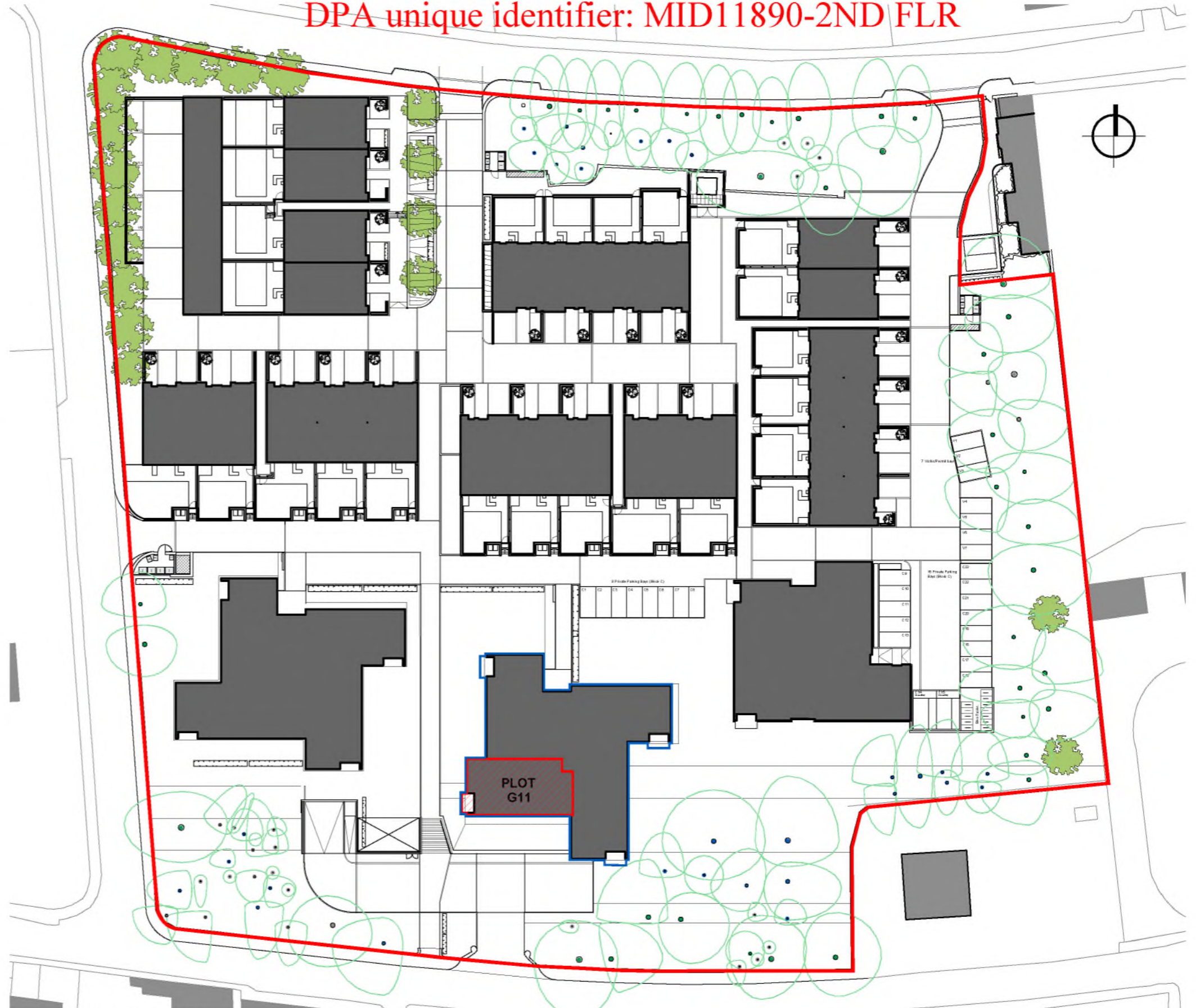
02 Plot G11 - Title Plan n.t.s
