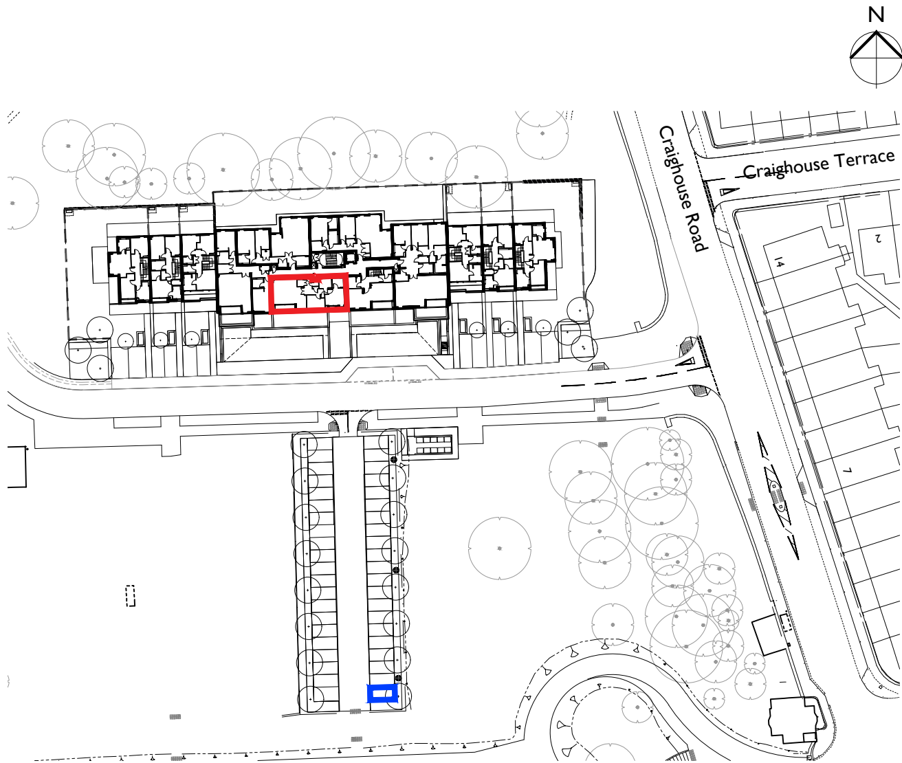
Deed Plan 1:1000
