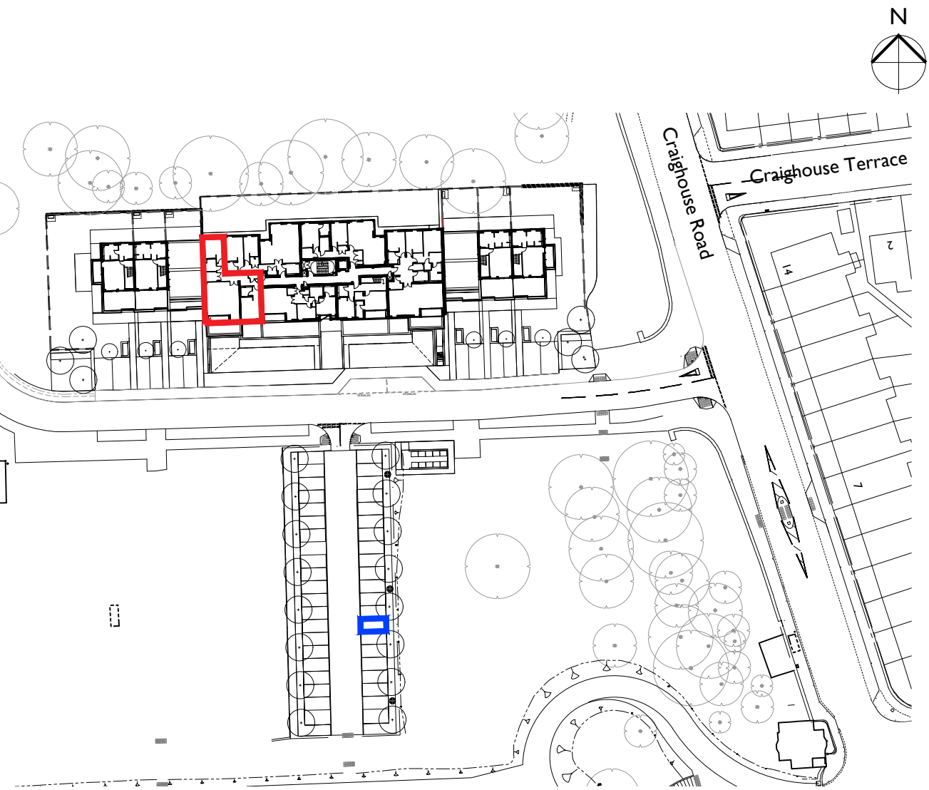
Deed Plan 1:1000
