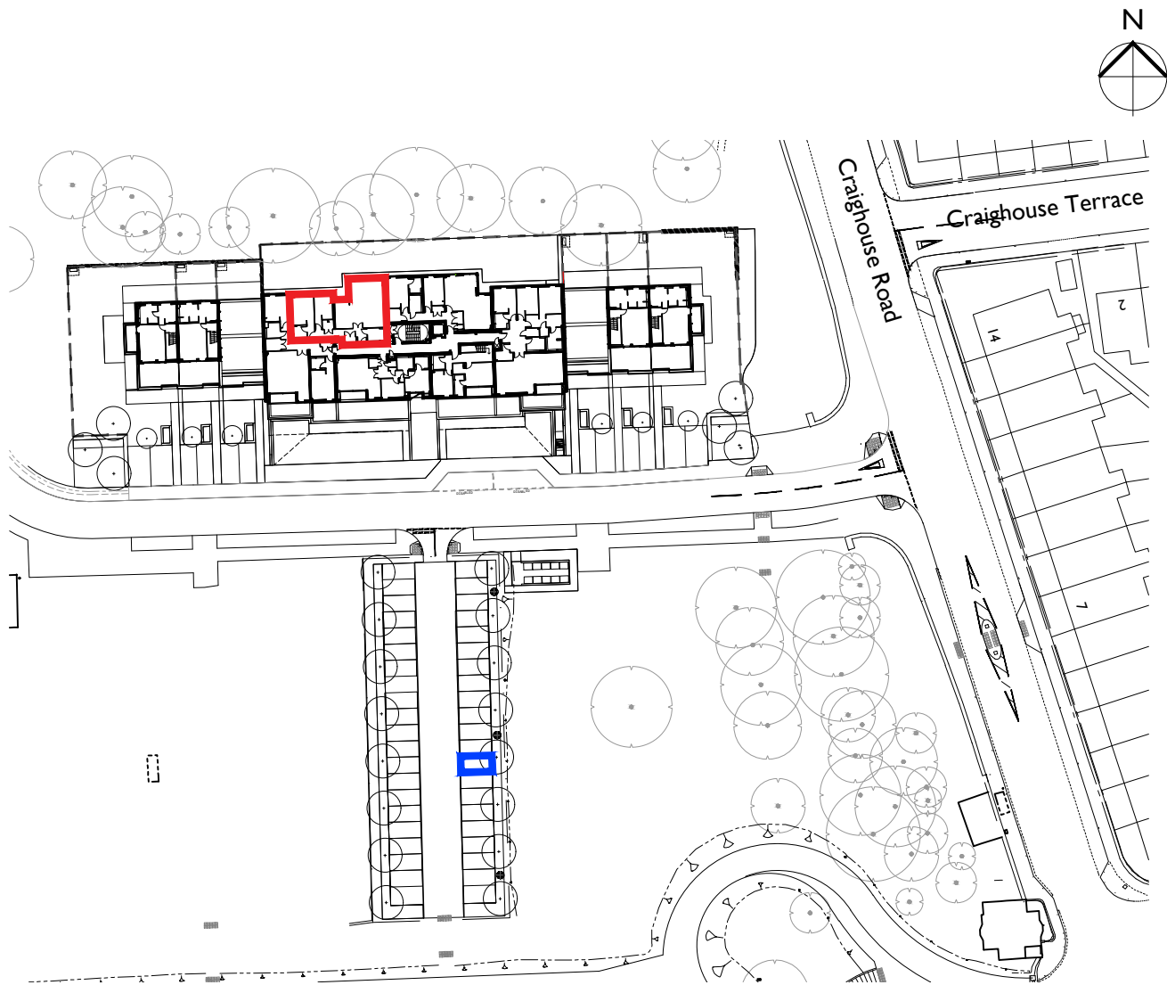
Deed Plan 1:1000
