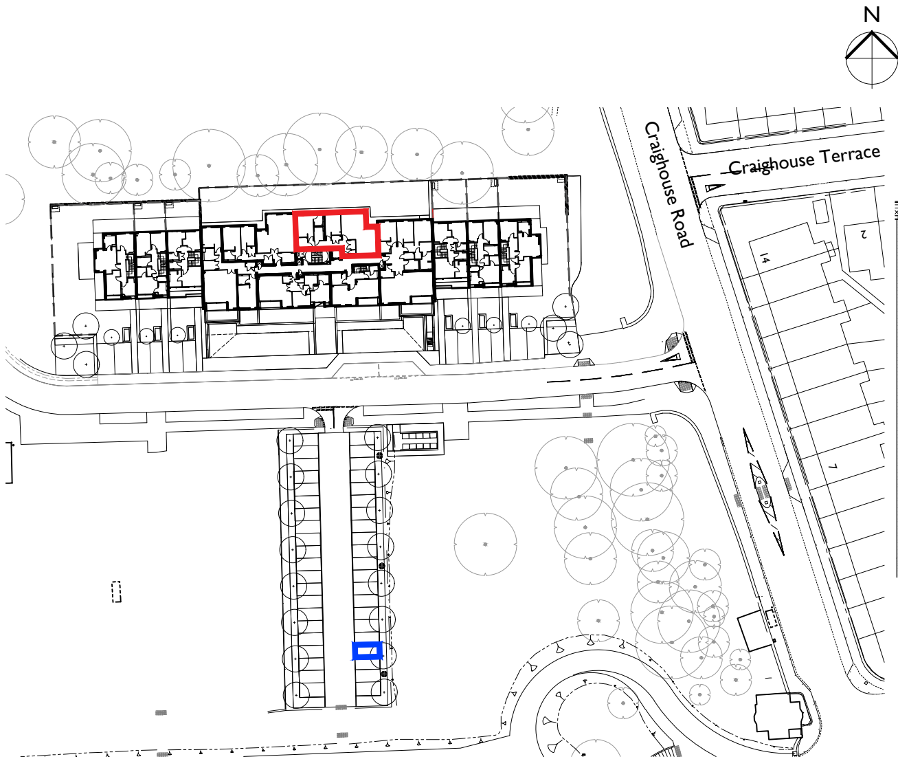
Deed Plan 1:1000
